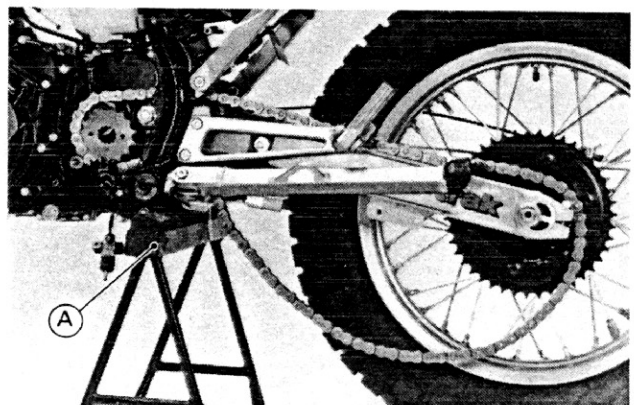
A. Abstützung
