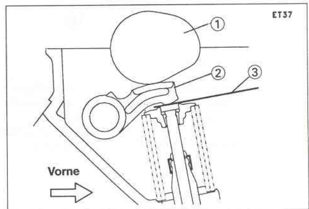
1. Nocken 2. Kipphebel
