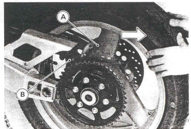
A. Hinterrad B. Hinterrad-Bremsattel und Bremsattelhalterung
