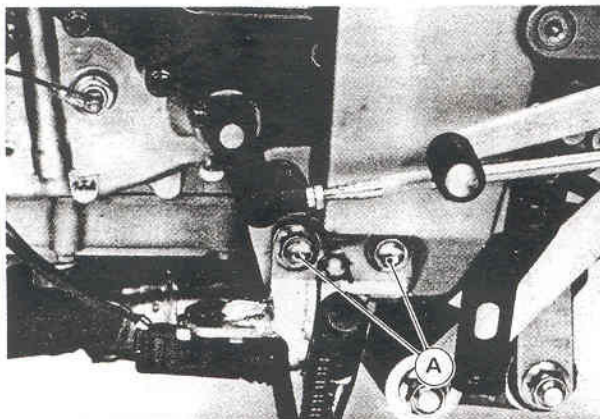
A. Schrauben für Seitenständer-Haltewinkel
