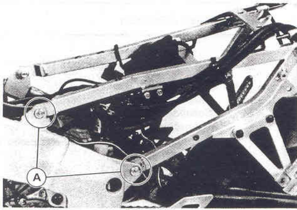
A. Schraube und Mutter für hinteren Rahmen
